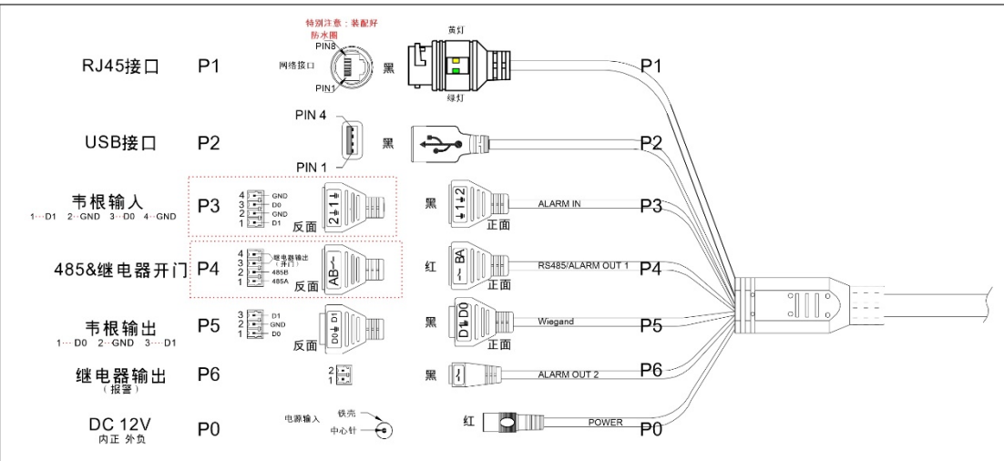
立装支架 7 头尾线
